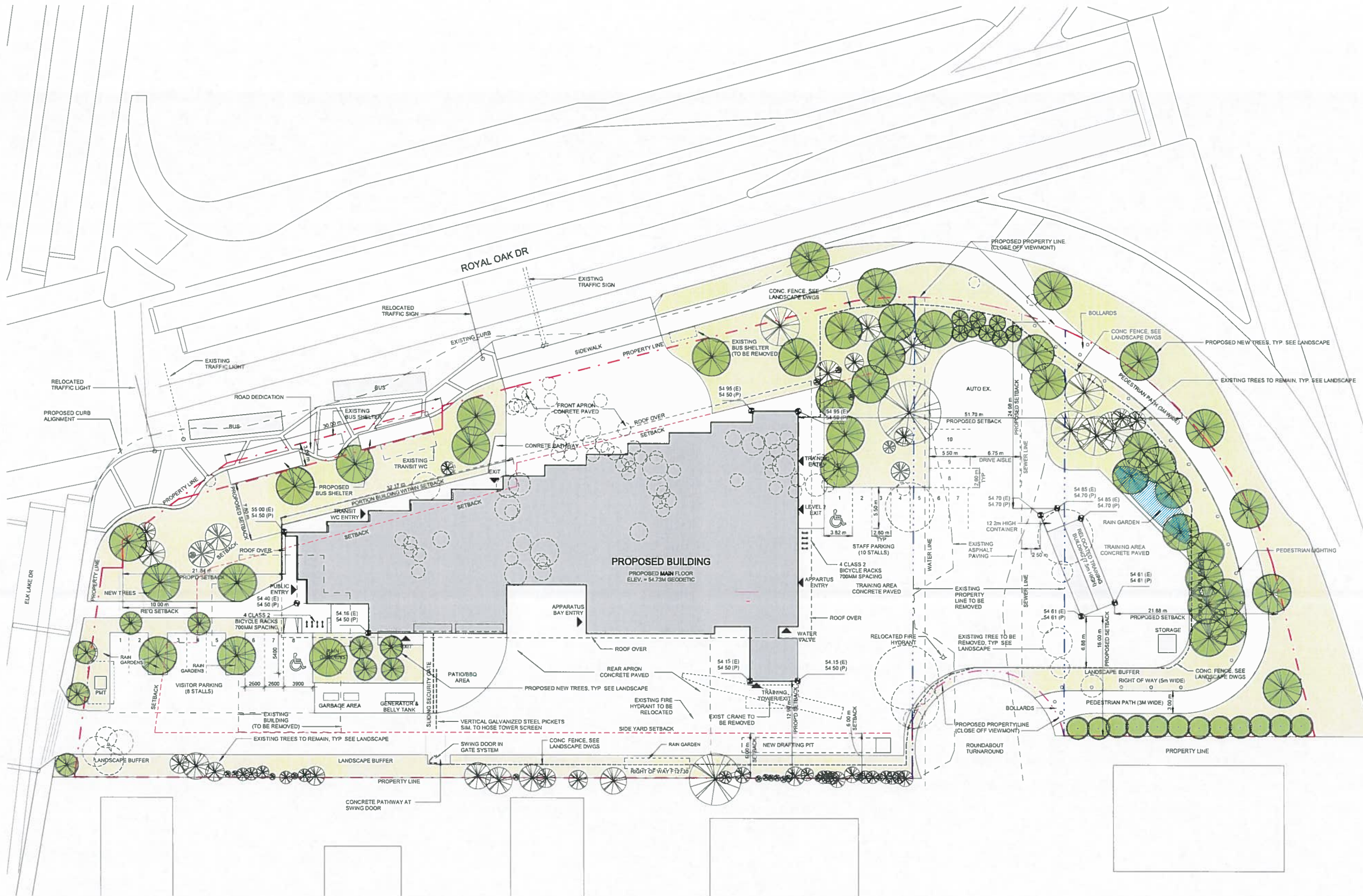
1 SITE PLAN 1:250
