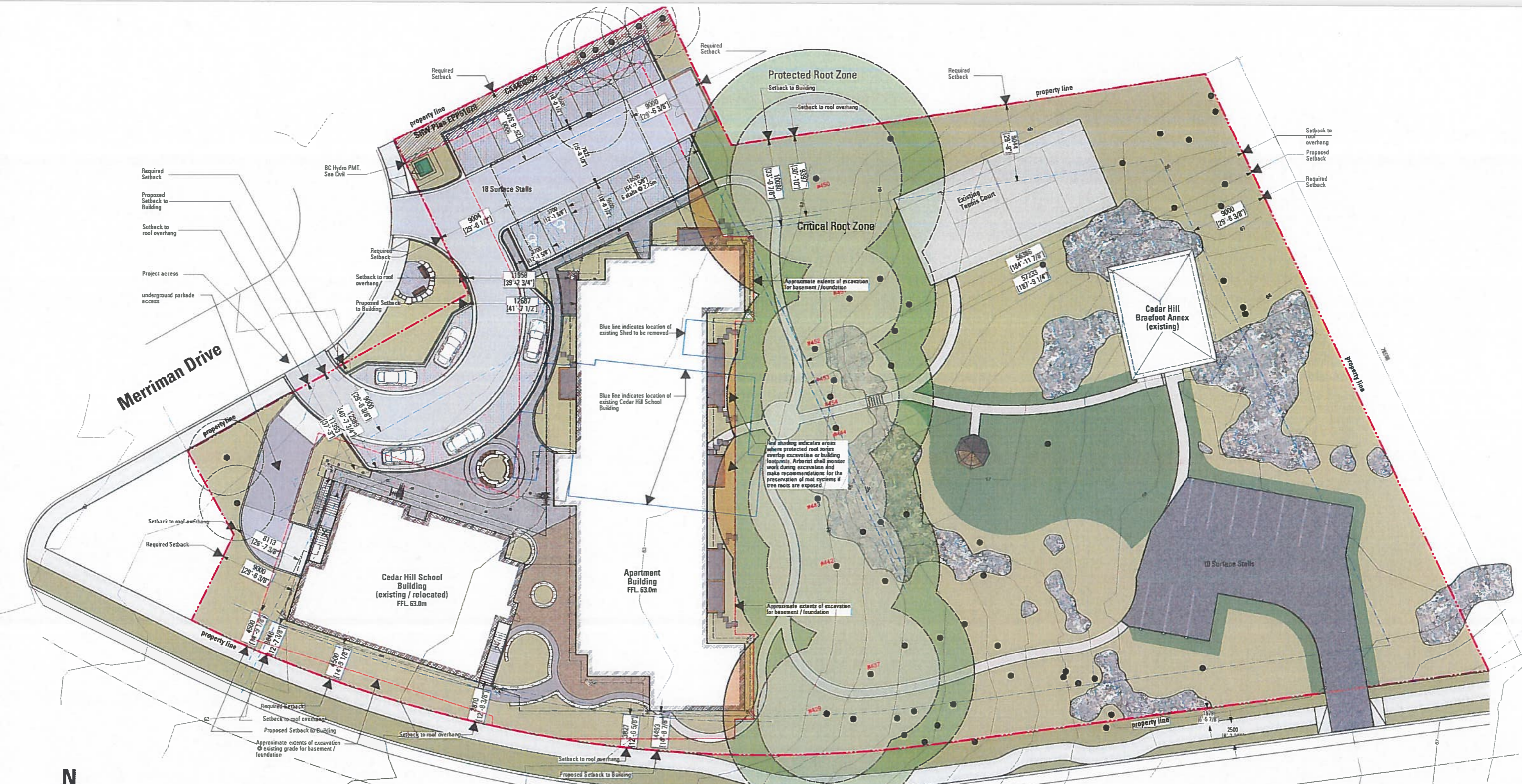
Site Plan Scale: 1:200m
