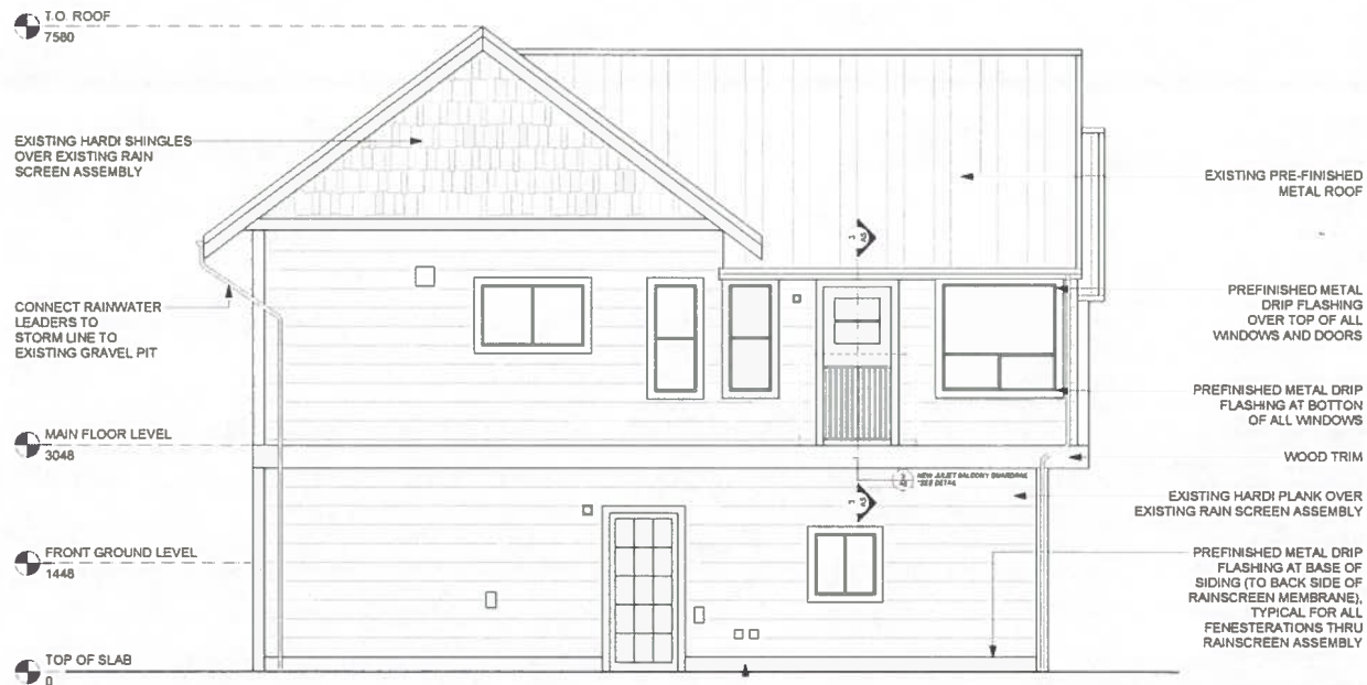
3 SOUTH ELEVATION A4 1:50
