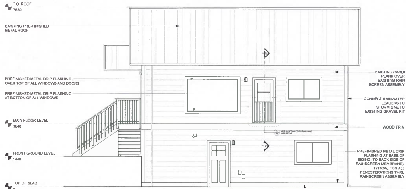
2 WEST ELEVATION A4 1:50
