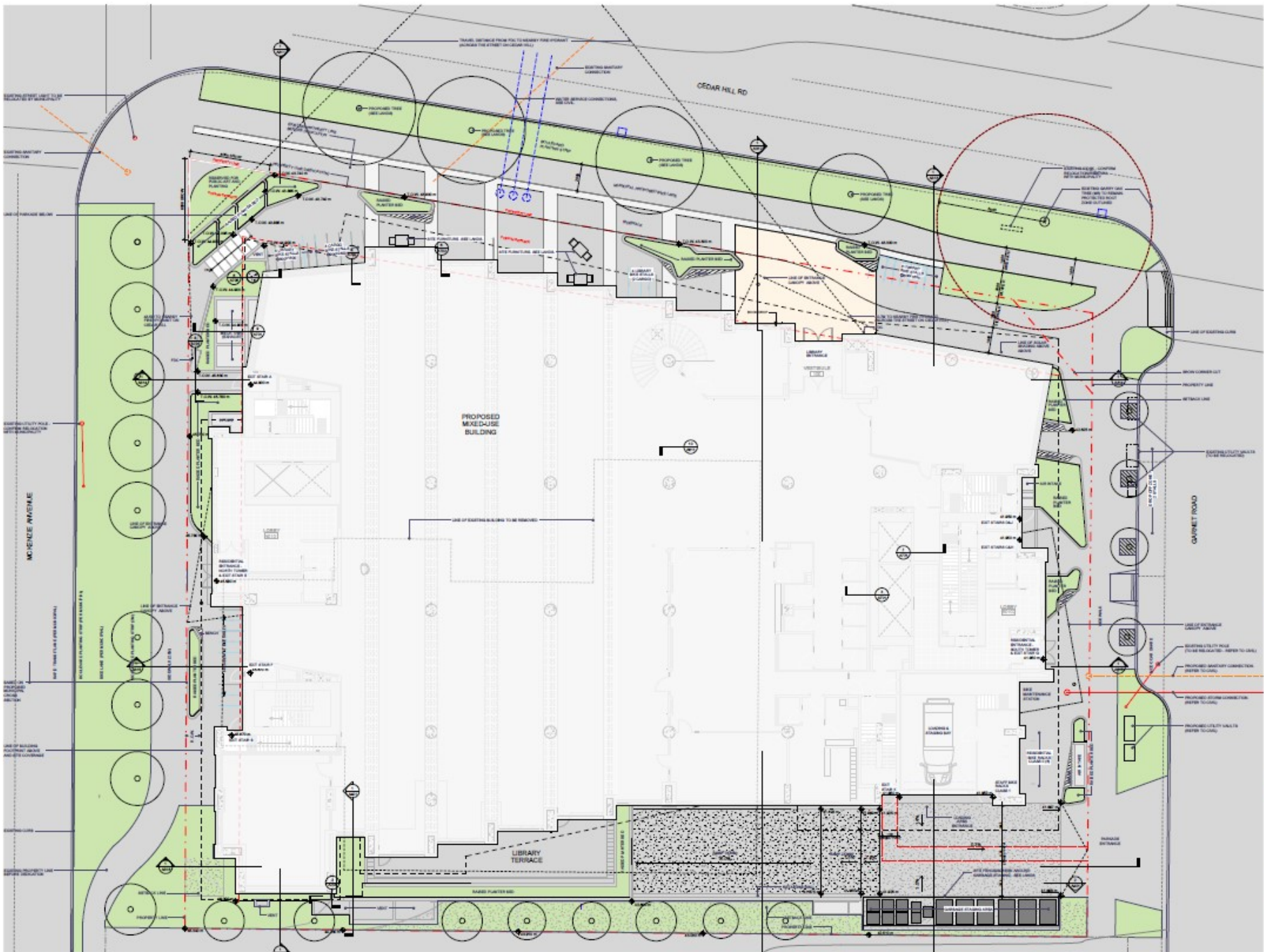
1 SITE PLAN 1/1/24
